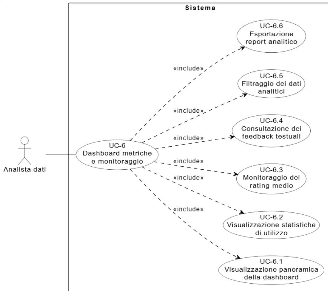
Figura 35: Diagramma del caso d'uso UC-6: Consulta metriche dell'AI Assistant
