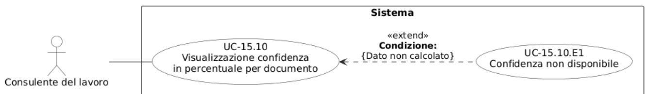
Figura 63: Diagramma del caso d'uso UC-15.10: Visualizzazione confidenza in percentuale per documento
