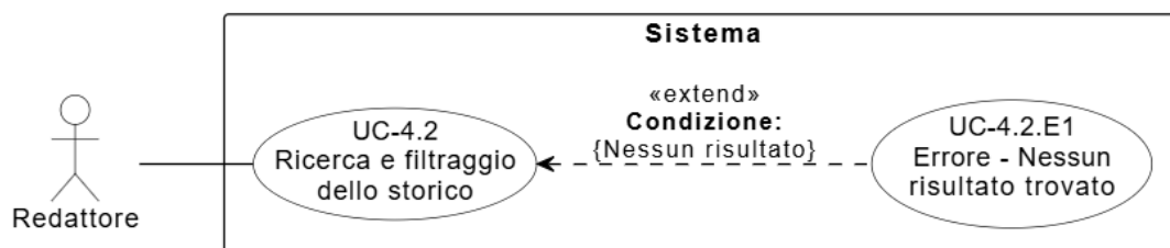
Figura 27: Diagramma del caso d'uso UC-4.2: Ricerca storico per parola chiave
