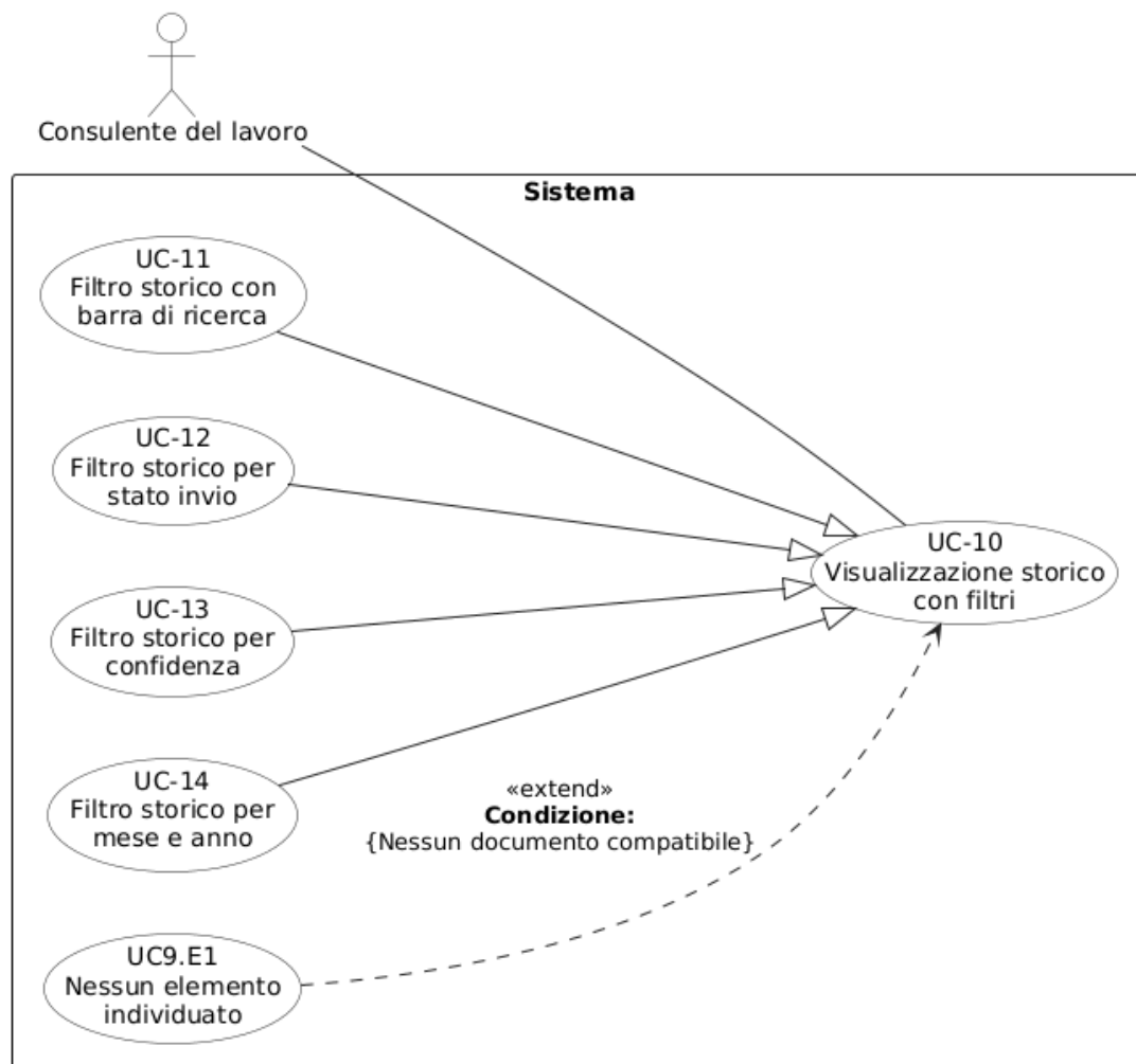
Figura 48: Diagramma del caso d'uso UC-10: Visualizzazione storico con filtri
