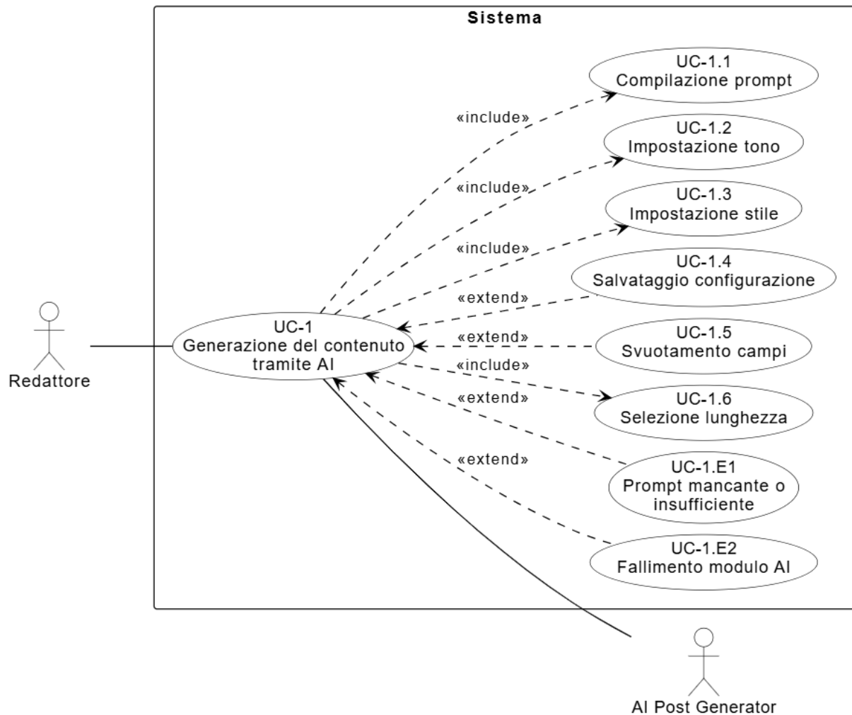
Figura 1: Diagramma del caso d'uso UC-1: Generazione del contenuto tramite AI
