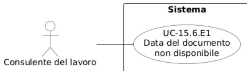
Figura 71: Diagramma del caso d'uso UC-15.6.E1: Data del documento non disponibile
