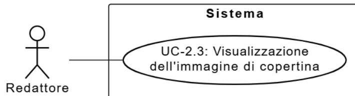
Figura 11: Diagramma del caso d'uso UC-2.3: Visualizzazione dell'immagine di copertina
