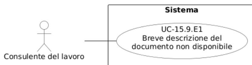
Figura 73: Diagramma del caso d'uso UC-15.9.E1: Breve descrizione del documento non disponibile
