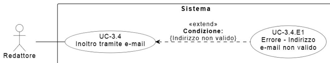
Figura 23: Diagramma del caso d'uso UC-3.4: Inoltra documento via e-mail
