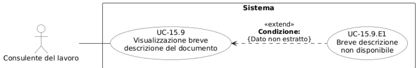
Figura 62: Diagramma del caso d'uso UC-15.9: Visualizzazione breve descrizione del documento
