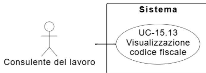
Figura 66: Diagramma del caso d'uso UC-15.13: Visualizzazione codice fiscale
