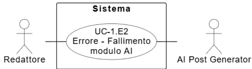
Figura 7: Diagramma del caso d'uso UC-1.E2: Errore per fallimento del modulo AI
