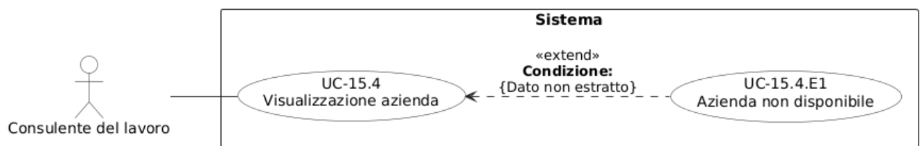
Figura 57: Diagramma del caso d'uso UC-15.4: Visualizzazione azienda
