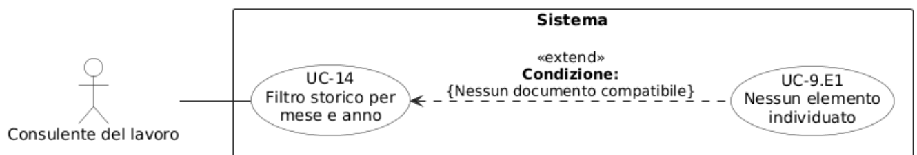
Figura 52: Diagramma del caso d'uso UC-14: Filtro storico per mese e anno
