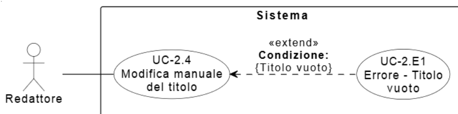
Figura 12: Diagramma del caso d'uso UC-2.4: Modifica titolo bozza
