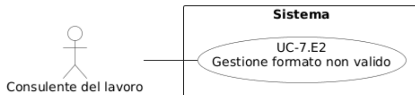
Figura 44: Diagramma del caso d'uso UC-7.E2: Gestione formato non valido
