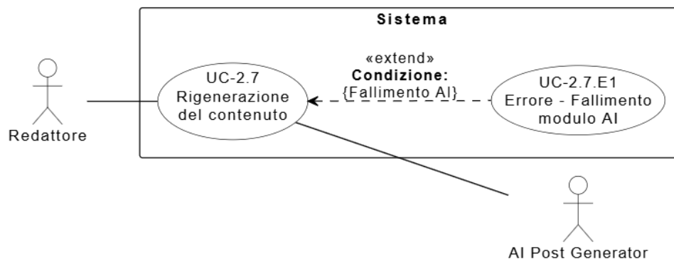
Figura 17: Diagramma del caso d'uso UC-2.7: Rigenera bozza
