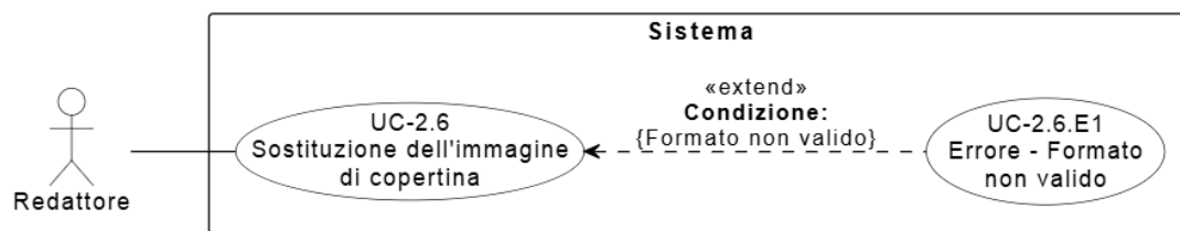
Figura 15: Diagramma del caso d'uso UC-2.6: Sostituisci immagine copertina
