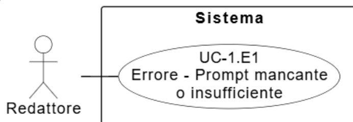
Figura 6: Diagramma del caso d'uso UC-1.E1: Errore per prompt mancante o insufficiente
