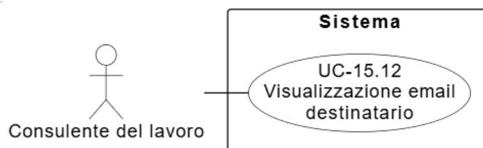
Figura 65: Diagramma del caso d'uso UC-15.12: Visualizzazione email destinatario
