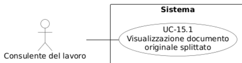
Figura 54: Diagramma del caso d'uso UC-15.1: Visualizzazione della porzione di documento relativa al dipendente
