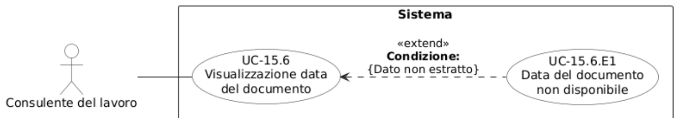
Figura 59: Diagramma del caso d'uso UC-15.6: Visualizzazione data del documento
